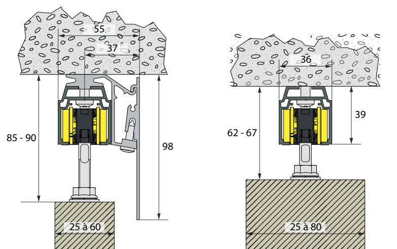
"shade screen" configuración sin bastidor. Grosor de la hoja: hasta 80 mm
