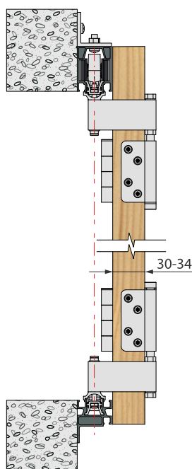
Montaje frontal del perfil guía
