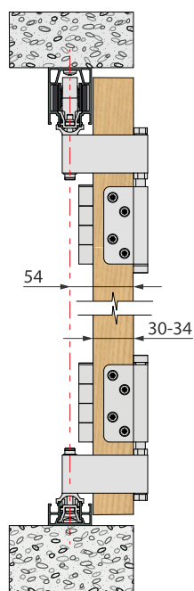
Ajuste de perfil guía
